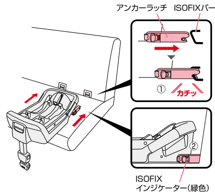
アンカーラッチ ISOFIXバー
