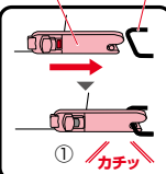
アンカーラッチ ISOFIXバー
