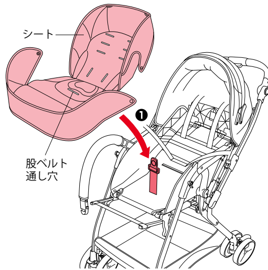
① 股ベルトをシートの通し穴に通す。
