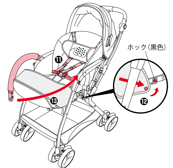
⑪ 肩ベルト、腰ベルトを股バックルに差し込む。 ⑫ フットガードのホックを本体座面の横側のベルトに付いているホック(黒色)にとめる。(左右) ⑬ フロントガードを取り付ける。
