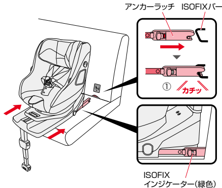
アンカーラッチ ISOFIXバー
